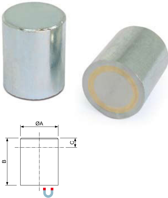
Passungstoleranz h6, kürzbar um Maß C
